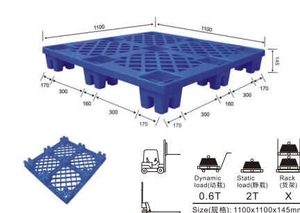
5#(concave) 9 Feet Pallet
